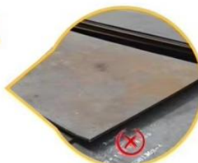
Others-No edge-mining
